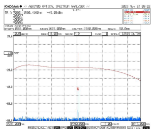
1590nm波长的小信号放大
