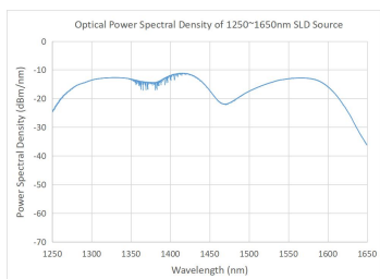
1250~1650nm波段SLD光源光谱 (1350~1400nm为OH-吸收峰)
