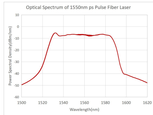
光谱(宽谱)
