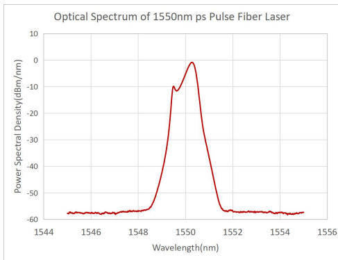
光谱(窄谱)
