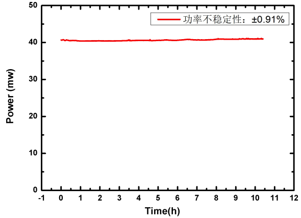
功率稳定性
